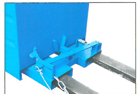
Hebel-Verschluss
